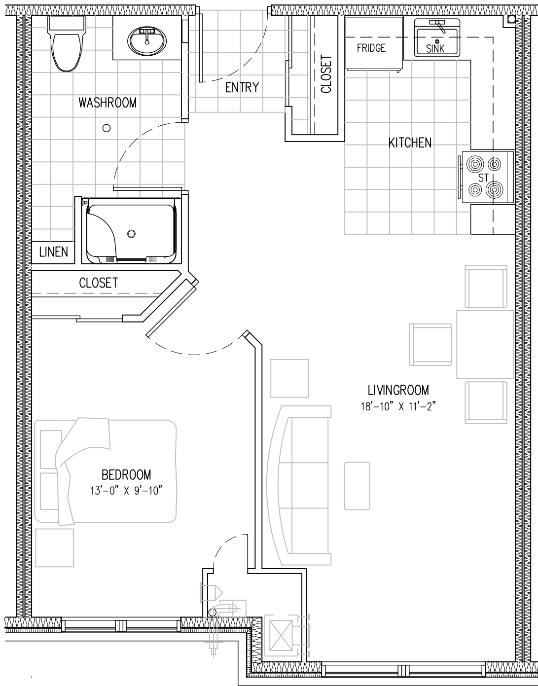
SUITE B 585.0 SQ. FT. (54.4 SQ. M.)
